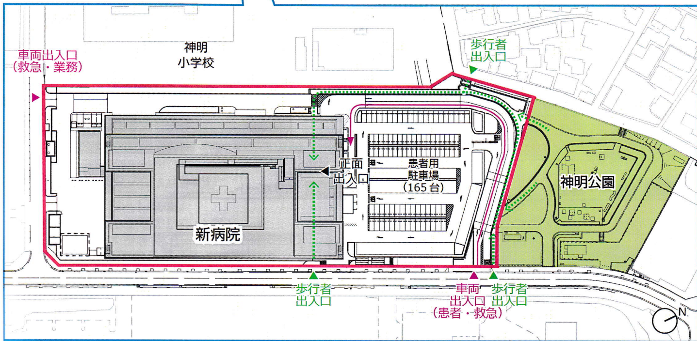
配置図
